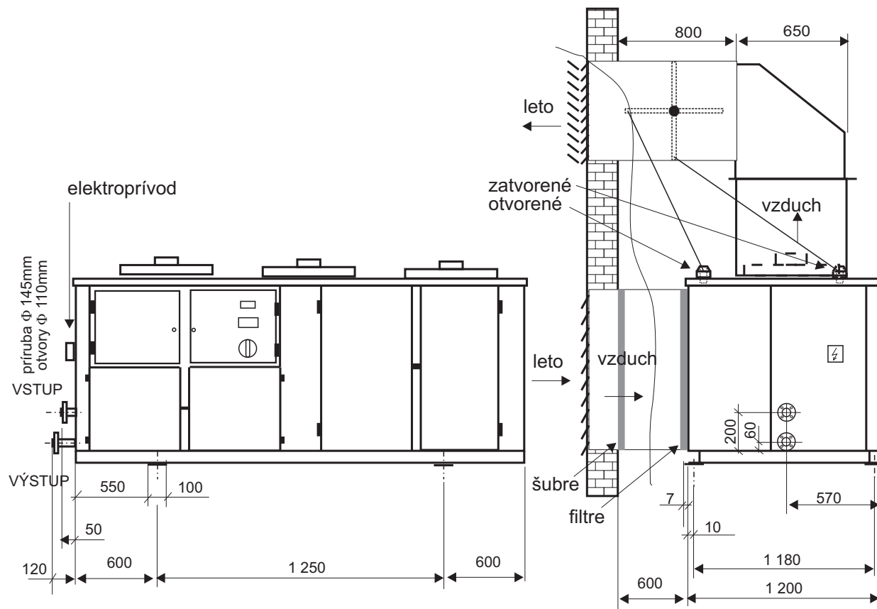
UMIESTNENIE CHLADIČA
