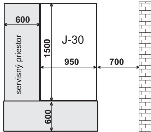
UPOLOHOVANIE CHLADIČA
