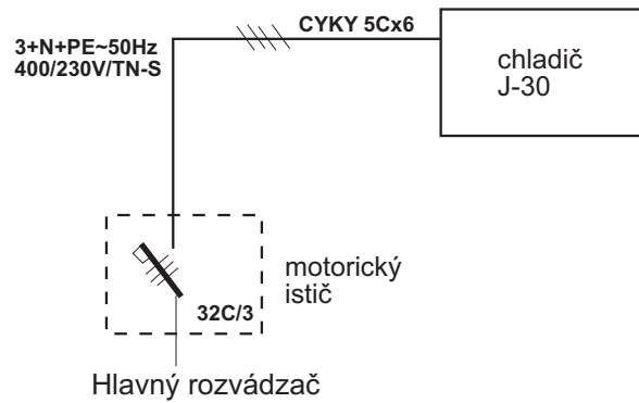
ELEKTRICKÉ ZAPOJENIE
