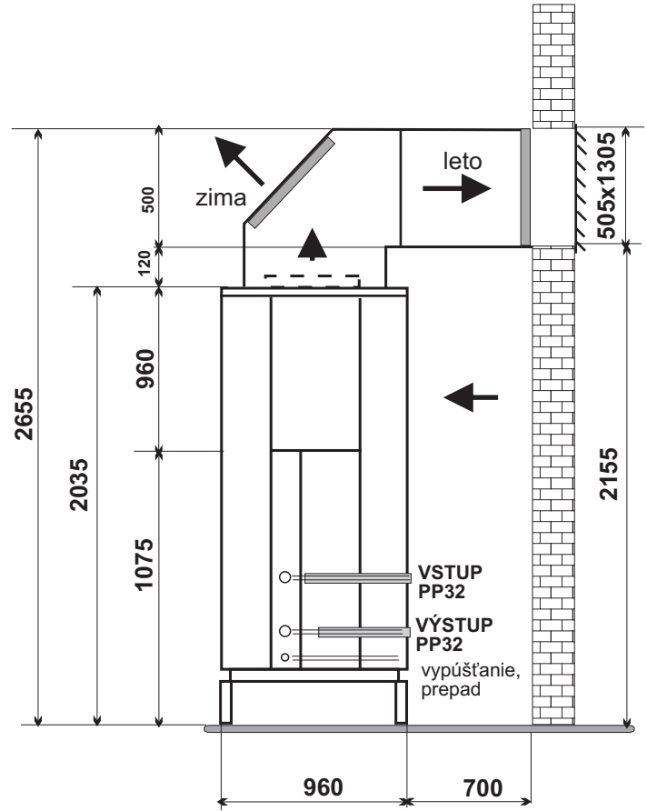
UPOLOHOVANIE CHLADIČA
